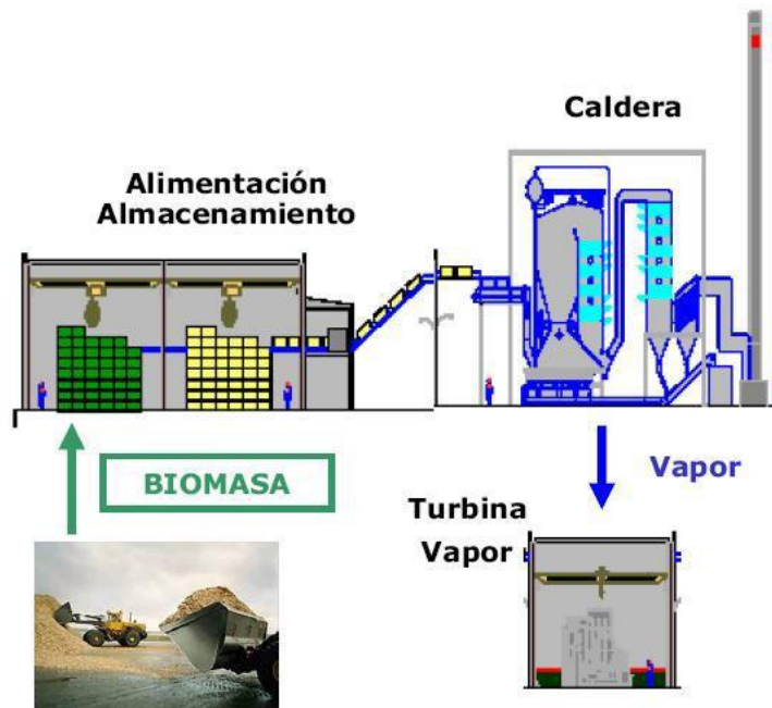
Ilustración 2, Esquema funcionamiento de una planta de biomasa
